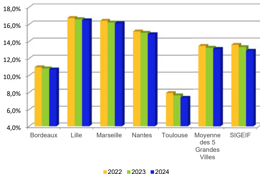
Part de réseau aérien dans le réseau total BT + HTA (en % de la longueur totale des réseaux)
